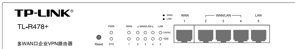
图 2-4 TL-R478+前面板示意图
